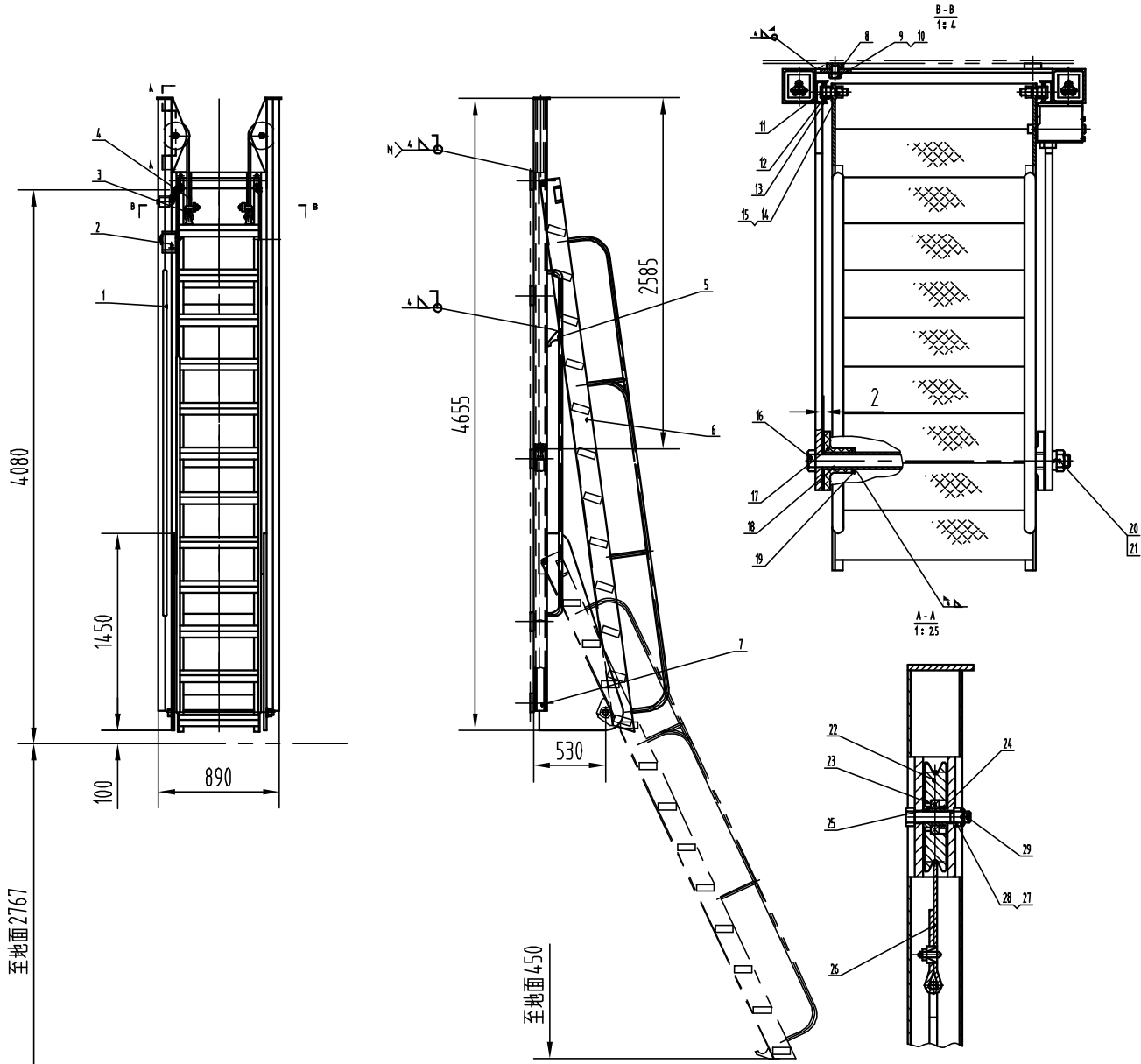
9.4. Лестница сдвижная (К1801.09.08.00)
